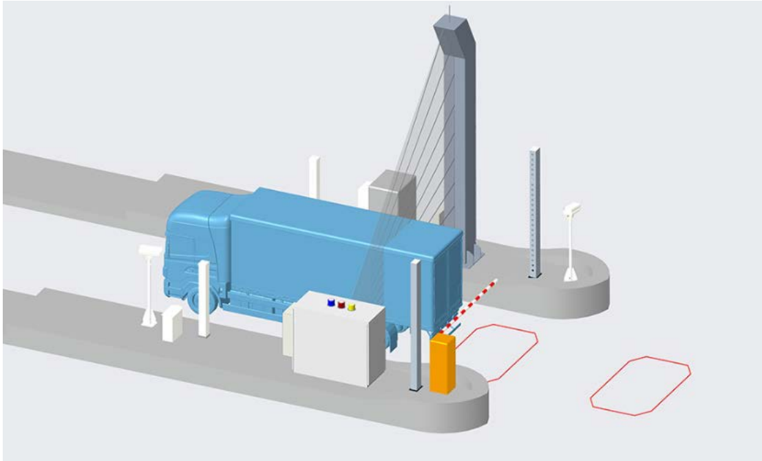
图 10 降杆过程
