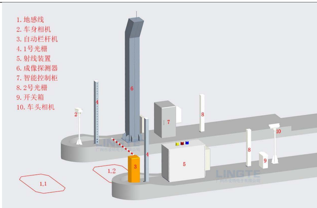
图 6 本项目绿通车辆快检系统示意图
